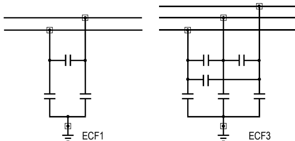
Figura 5.1: Filtri ECF
