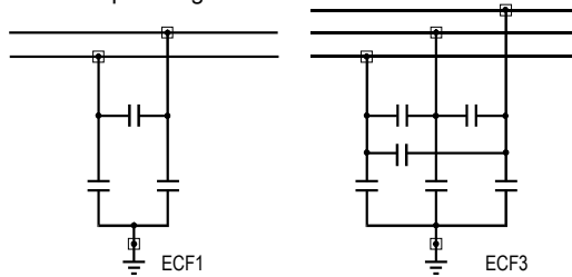
Abbildung 5.1: ECF Filter
