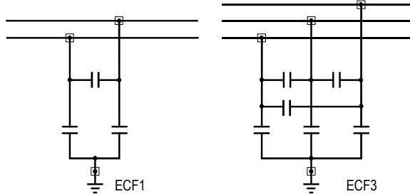
Figura 5.1: Filtros ECF
