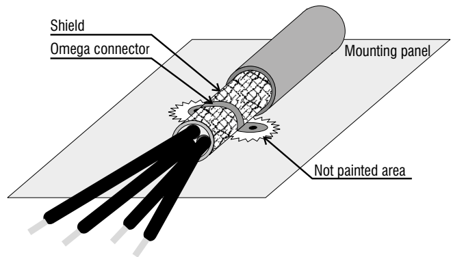
Figure 6.4: Connecteur de type OMEGA: mise à terre à 360° d'un câble blindé.
